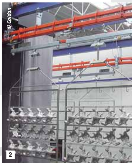
2 Overhead conveyor - operating in Germany. Trasportatore a soffitto in funzione in Germania.
