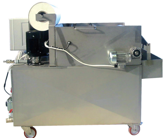
CCI000 - mobile Reinigungseinheit
