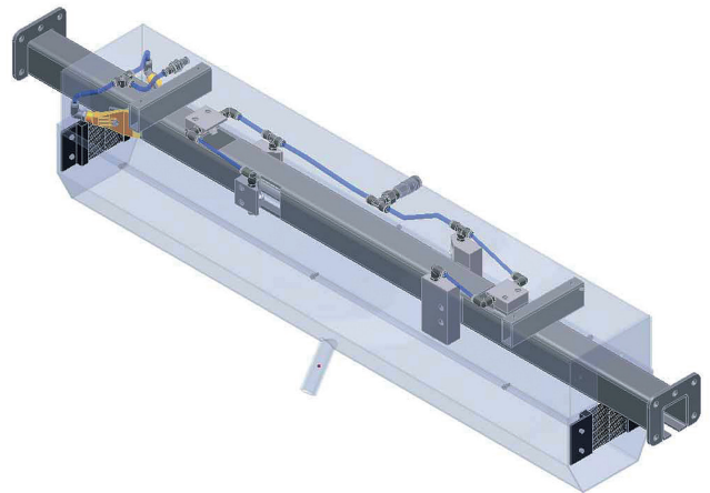
CCI000 - fest eingebaute Reinigungsprofil
